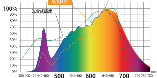
植物育成用ライト分光分布図
